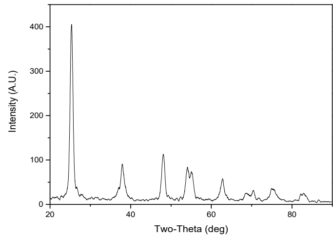
图3.1 催化剂的XRD图谱（宋体加粗小四号）
